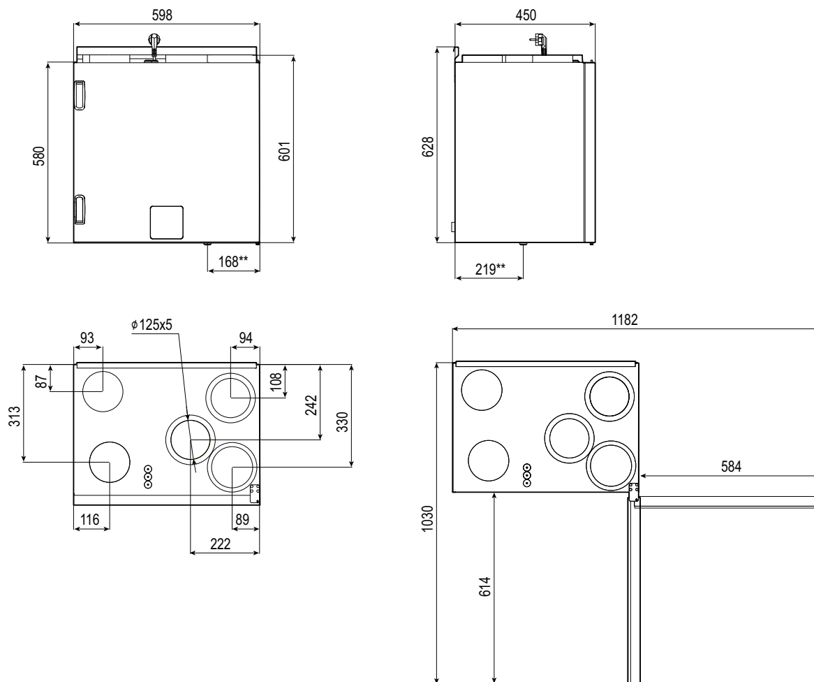
Pav. 2 Kairinio įrenginio matmenys
