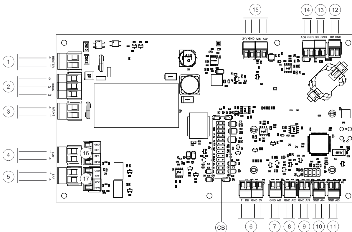
Pav. 5 Pagrindinės plokštės jungtys
