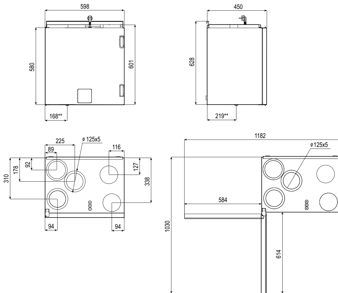
Pav. 3 Dešinio įrenginio matmenys
